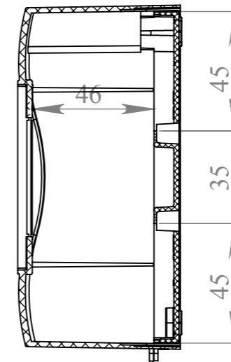
СЕЧЕНИЕ А-А
